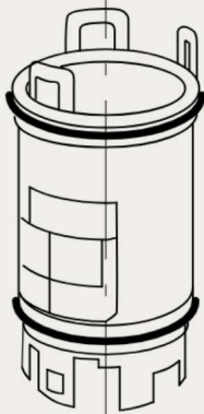
Vedení vody Rozhraní k tělesu armatury, reguluje přívod a výdej vody
